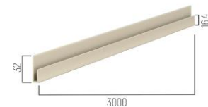
Стартовый профиль
