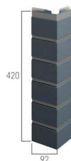
Угол наружный
