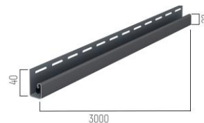
J профиль
